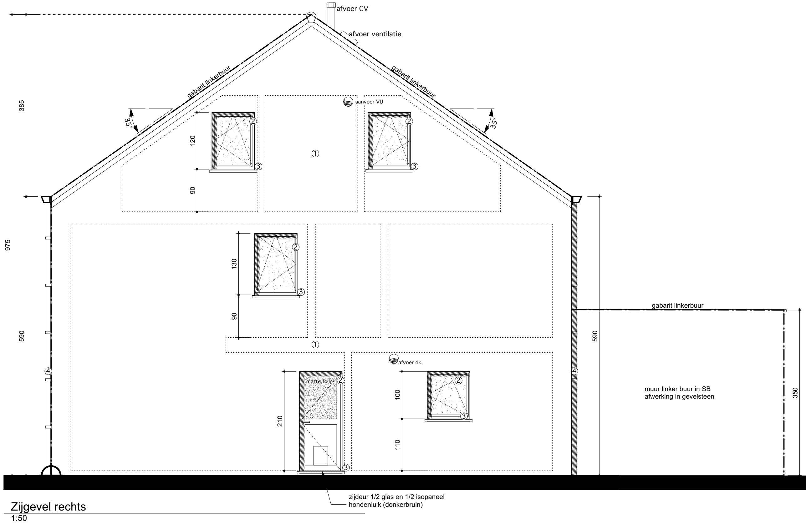
Voorgevel 1:50
