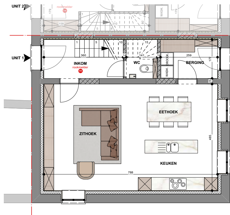
GELIJKVLOERS OPP.: 68,62m 2
