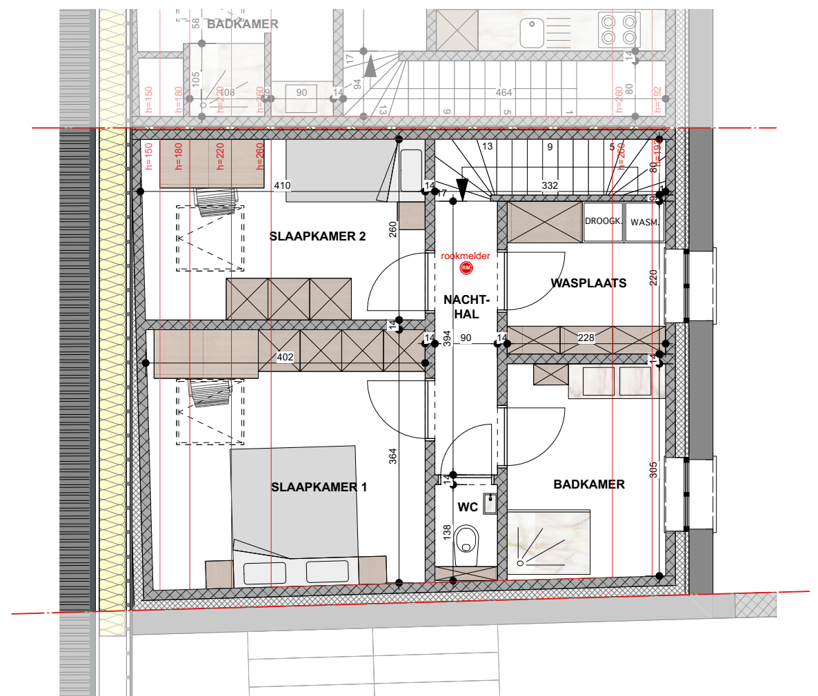
VERDIEPING OPP.: 61,02m 2
