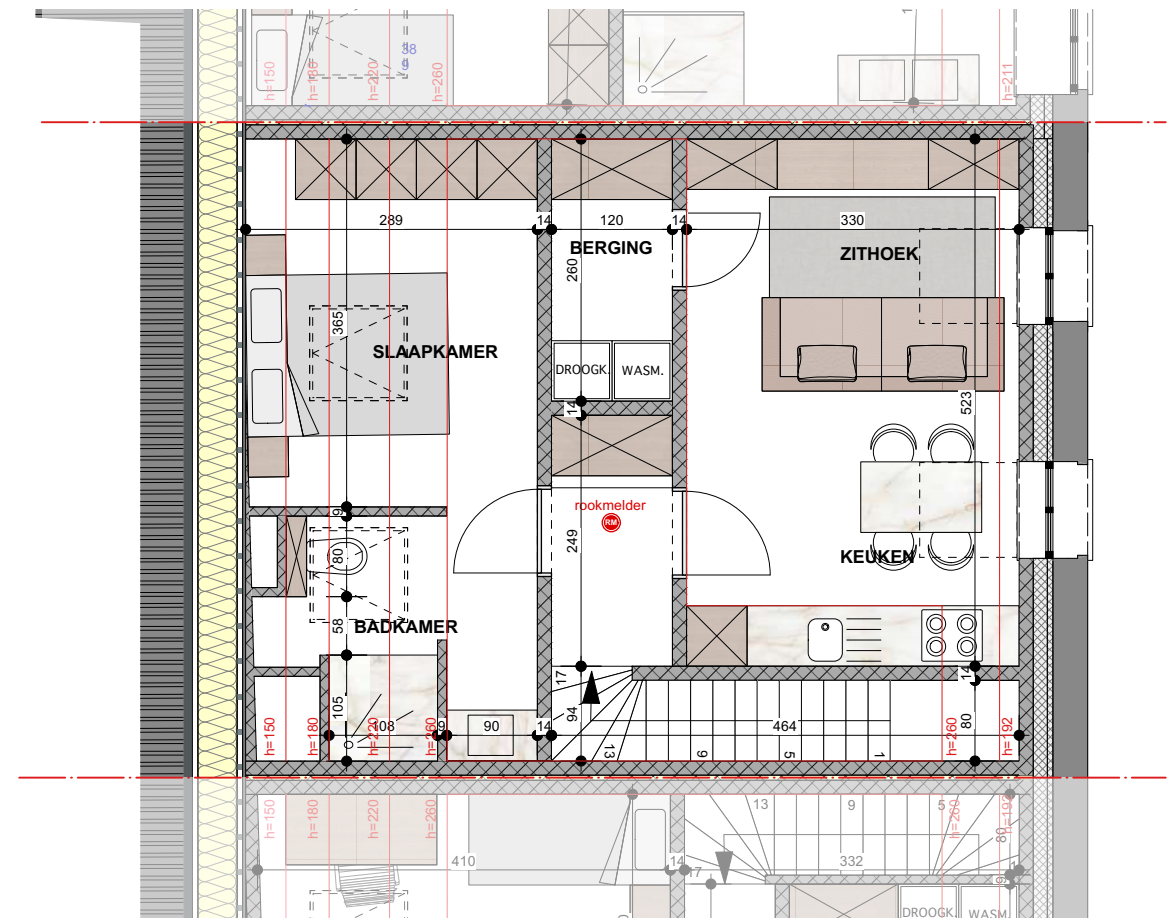
VERDIEPING OPP.: 61,10m 2
