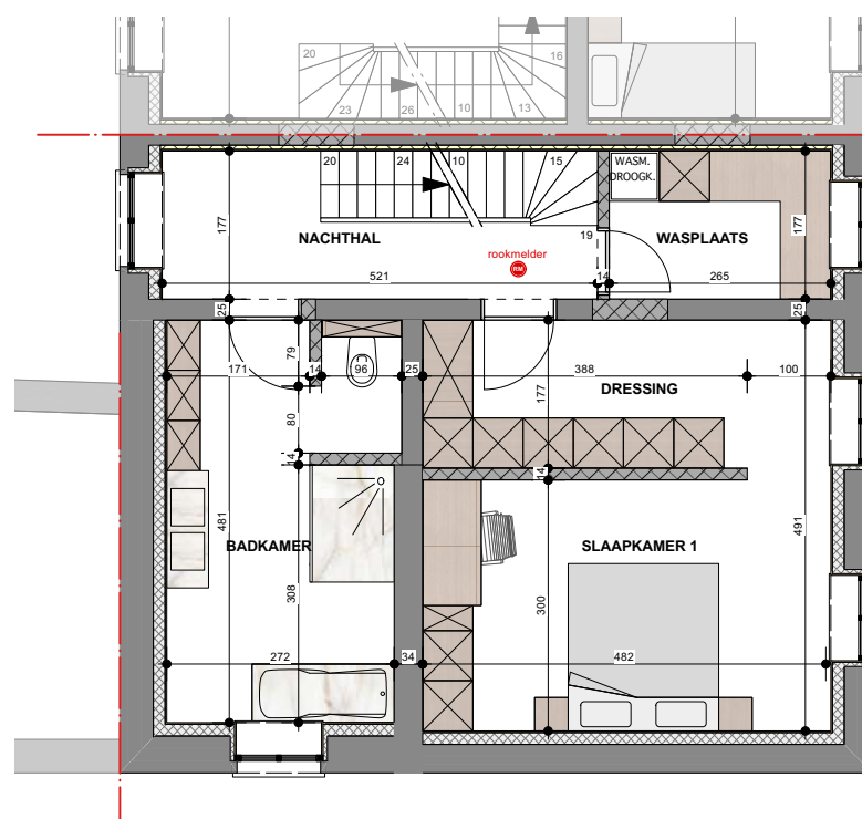
VERDIEPING +1 OPP.: 68,62m 2
