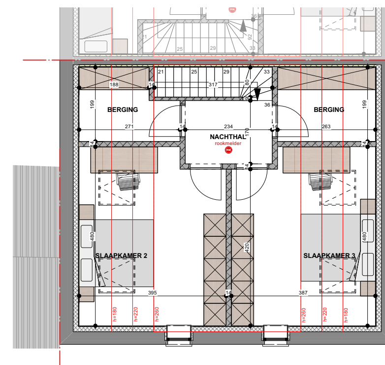
VERDIEPING +2 OPP.: 68,62m 2
