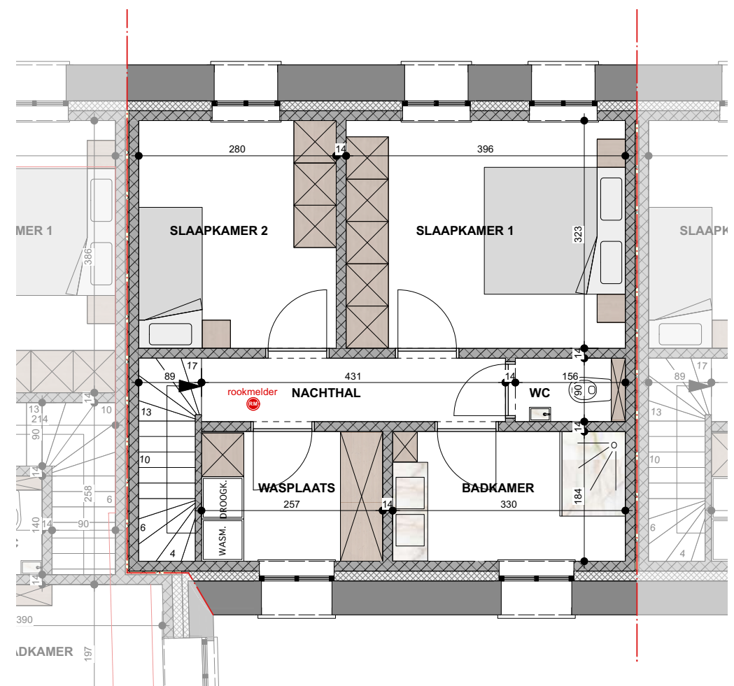
VERDIEPING OPP.: 55,79m 2
