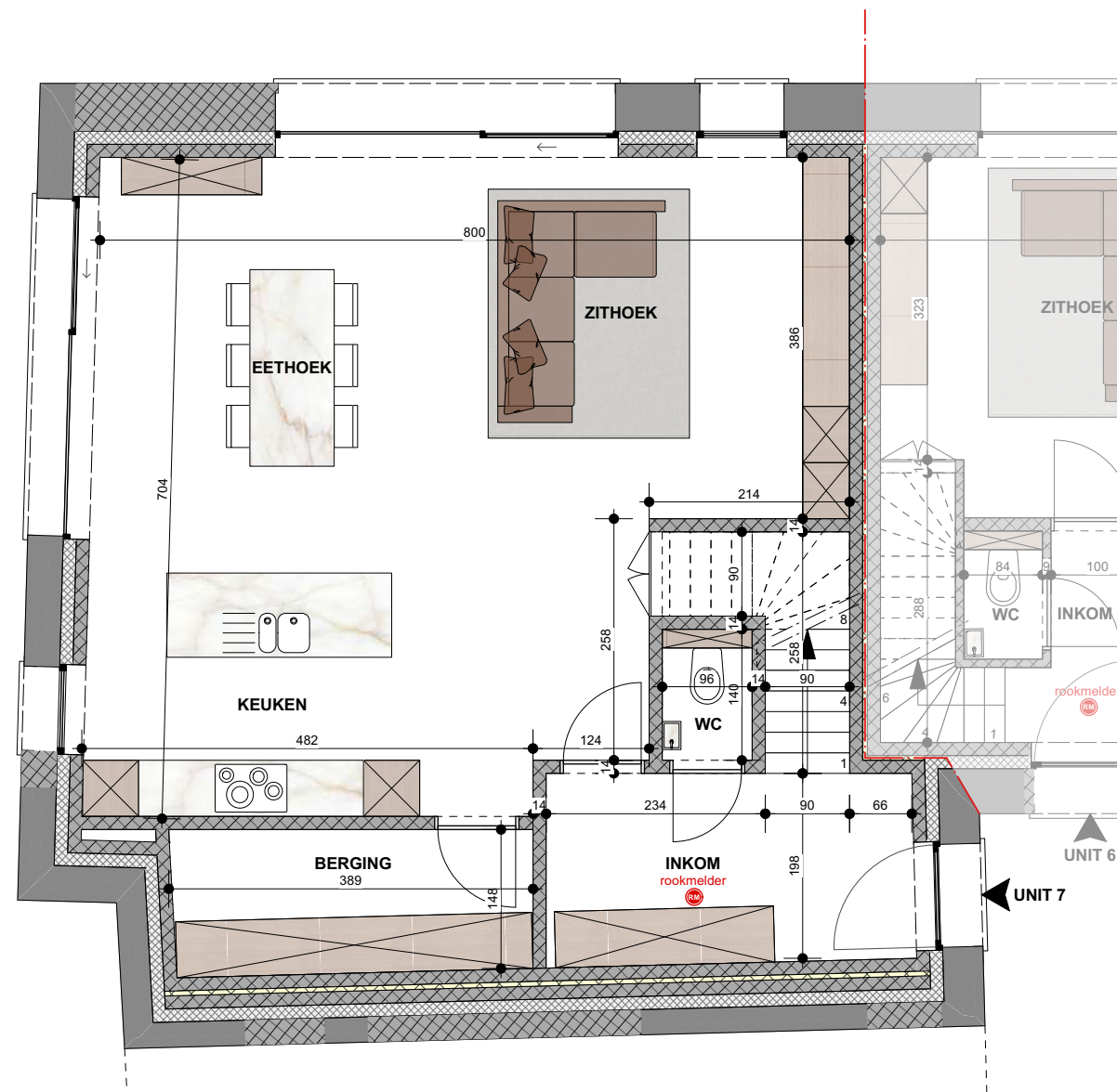
GELIJKVLOERS OPP.: 93,13m 2
